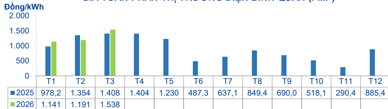
GIÁ TOÀN PHẦN THỊ TRƯỜNG ĐIỆN BÌNH QUÂN (FMP)
