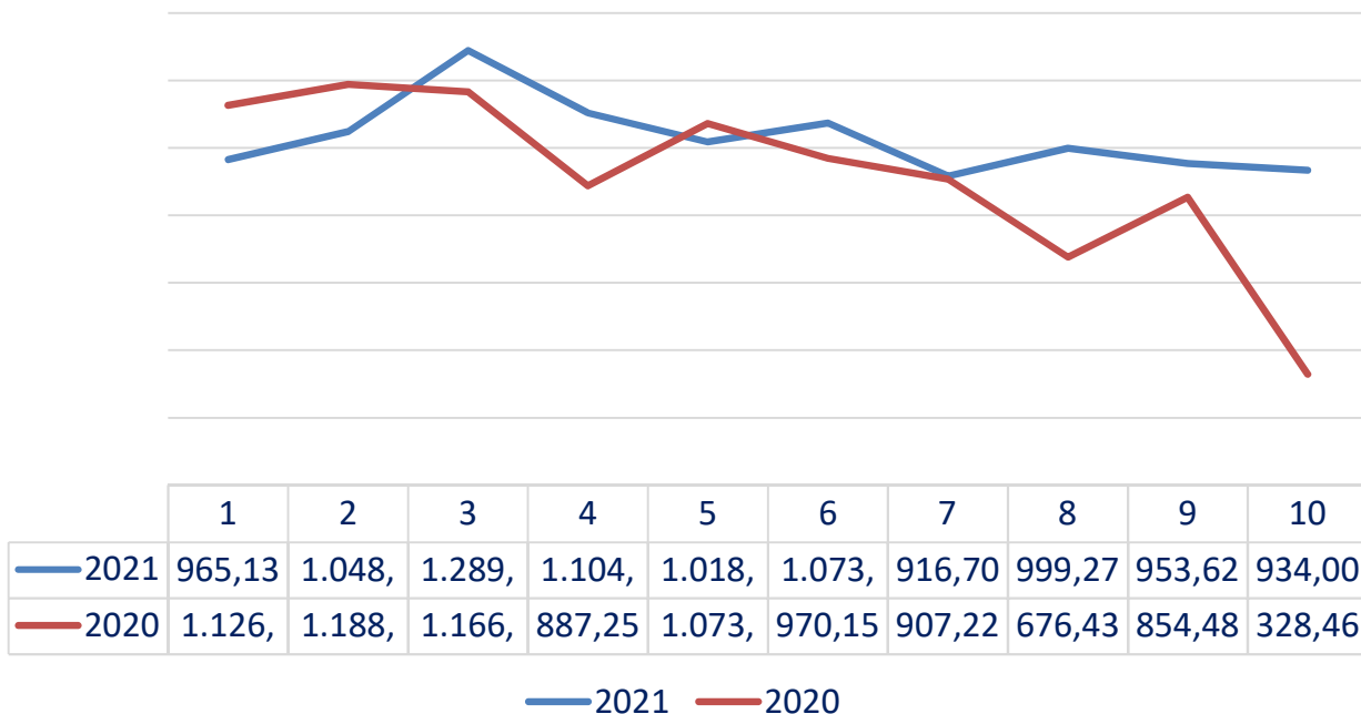
Giá toàn phần thị trường điện (FMP) bình quân tháng 1-10/2020 & 2021 (VND/kWh)
