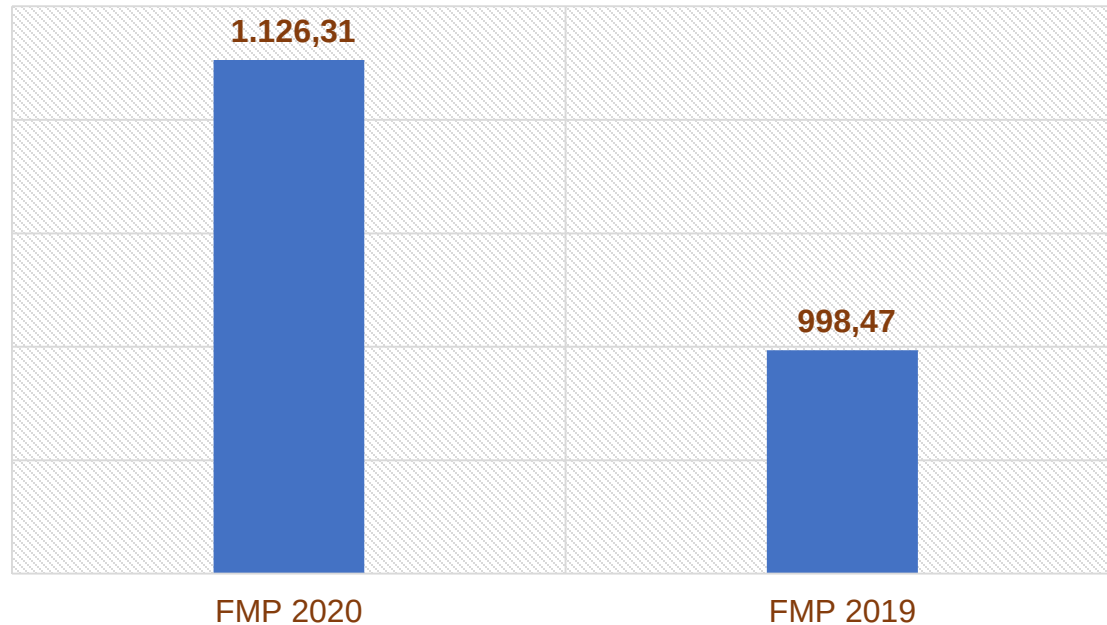
GIÁ TOÀN PHẦN THỊ TRƯỜNG ĐIỆN BÌNH QUÂN THÁNG 1 - FMP (VND/kWh)
